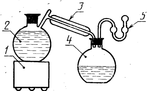
1 — электроплитка; 2 — дистилляционная колба; 3 — холодильник; 4 — колба-приемник; 5 — предохранительная воронка
